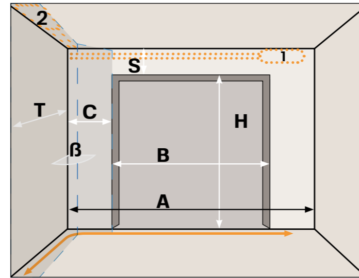
1 Sturzmontage 2 Seitenmontage Wenn Maß C größer als 700 mm nur Sturzmontage möglich.
